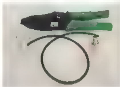
Alle onderdelen voor een pigtail RP SMA naar male-N met connector krimptang.
